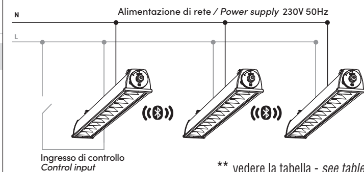
Schema applicativo per ingresso ausiliario di controllo Application diagram for auxiliary control input
