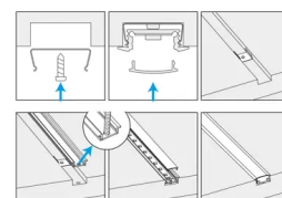
Esempio di installazione a incasso con clip
